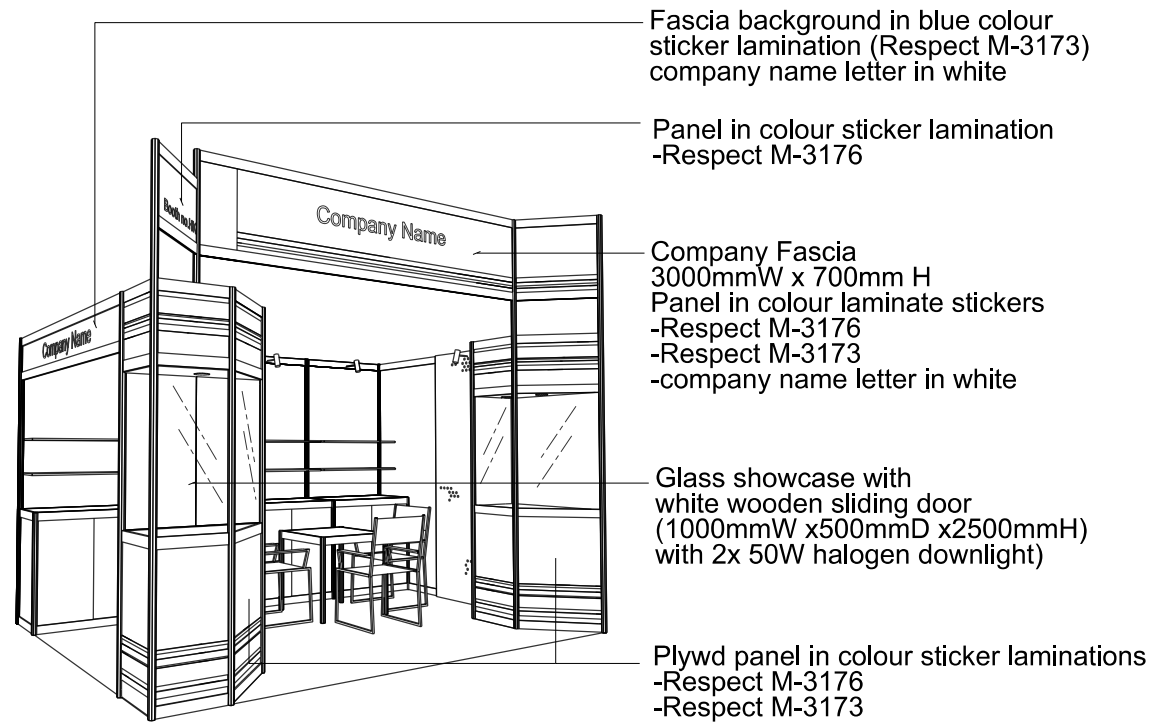
PERSPECTIVE N.T.S
