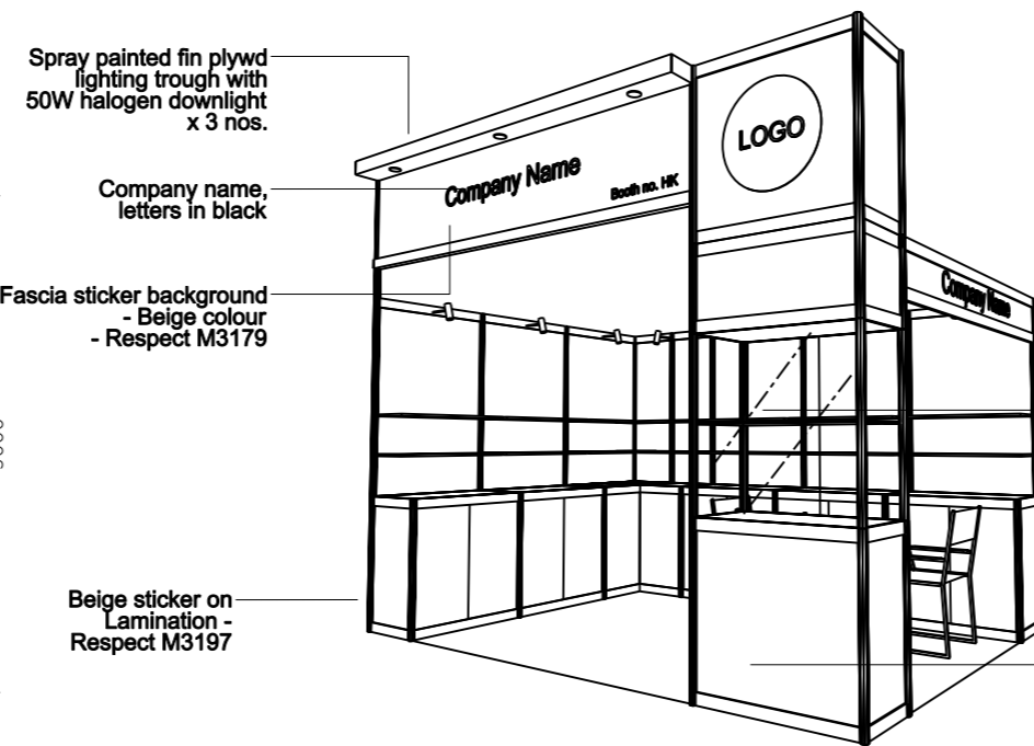
PERSPECTIVE N.T.S.
