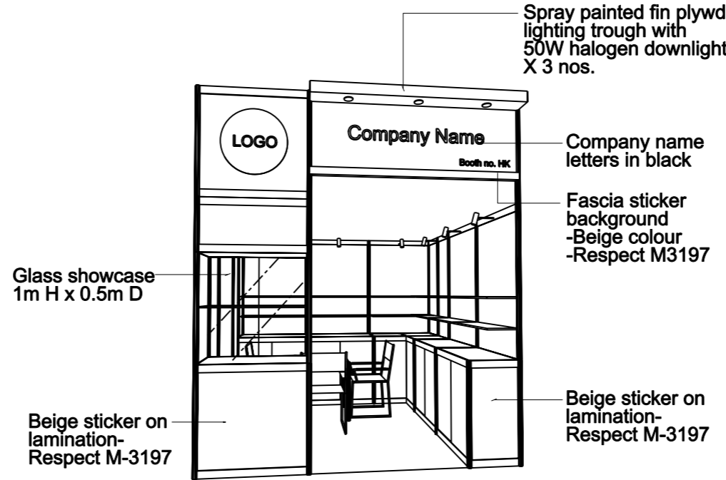
PERSPECTIVE N.T.S
