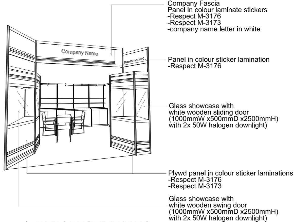
PERSPECTIVE N.T.S
